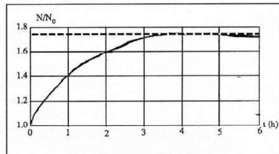
Figure 2 : Concentration des sels facilement solubles dans l'eau circulée pendant l'ajout continu d'eau d'appoint.
