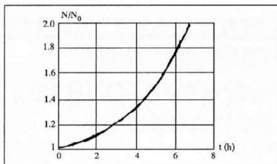
Figure 3 : Concentration des sels difficilement solubles dans l'eau circulée pendant l'ajout continu d'eau d'appoint.
