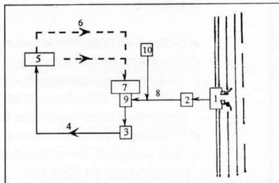
Figure 1 : Schéma d'adduction d'eau de circulation.
